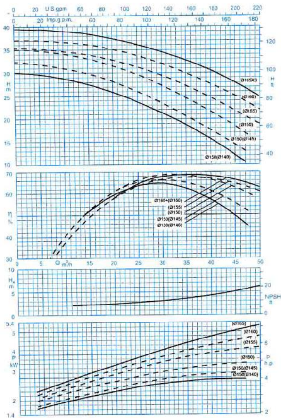
دور موتور ۲۹۰۰ / 2900 rpm For 1 Stage / منحنی یک طبقه
